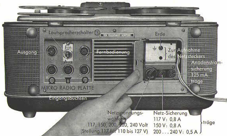
Rückansicht des Tonbandkoffers TK 35
